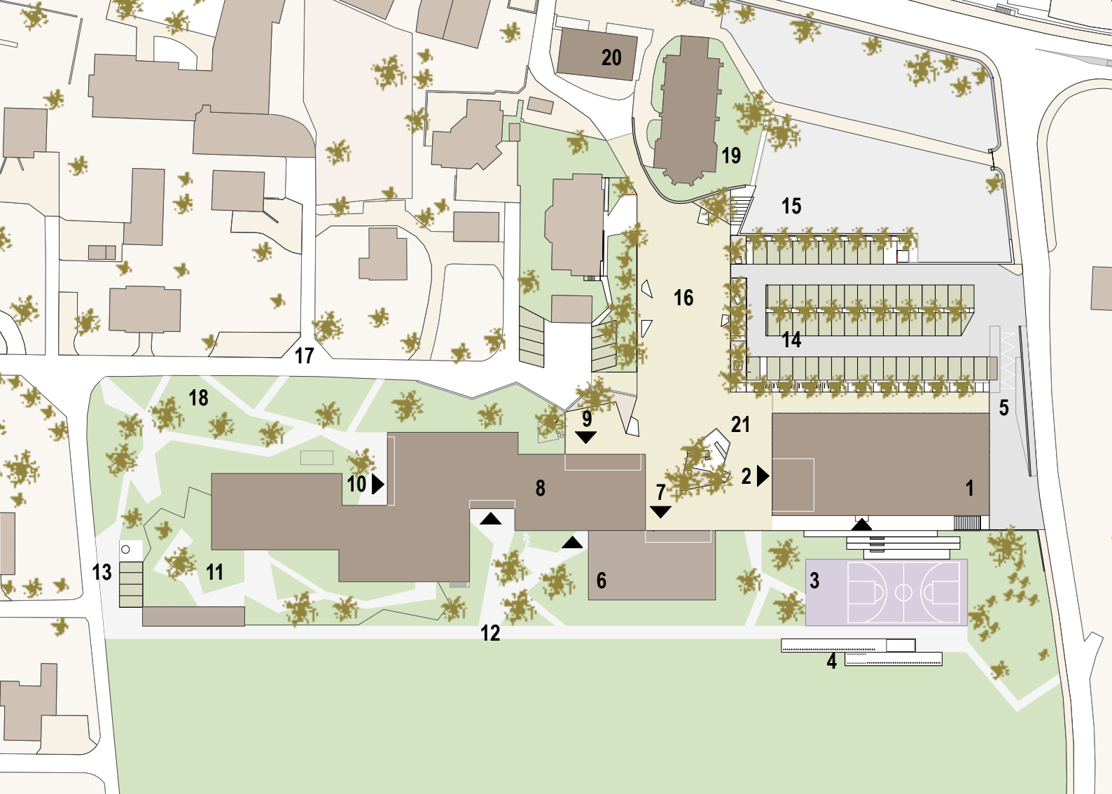
plan de situation_aménagement extérieurs__
